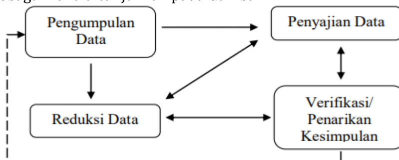
Gambar 1. Desain Analisis data Penelitian
