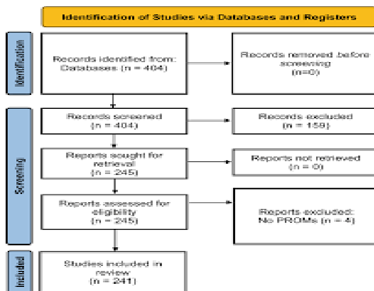
Gambar 1. Tahapan PRISMA
